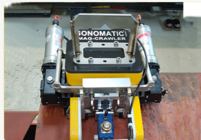
MAG-CRAWLER
